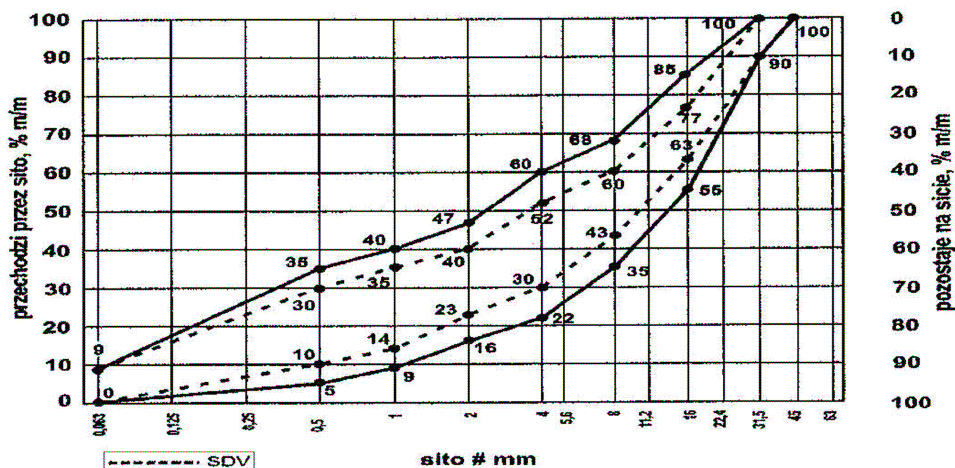
Rys. 2 Mieszanka niezwiązana 0/31, 5 do warstw podbudowy zasadniczej
