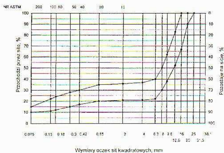
Rys. 2. Krzywe graniczne uziarnienia mieszanki mineralnej BA od 0 do 20 mm (mieszanka o nieciągłym uziarnieniu) do warstwy ściernalnej nawierzchni drogi o obciążeniu ruchem od KR3 do KR6
