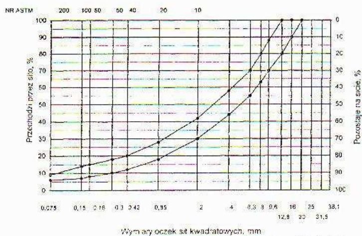
Rys. 3. Krzywe graniczne uziarnienia mieszanki mineralnej BA od 0 do 16 mm do warstwy ściernalnej nawierzchni drogi o obciążeniu ruchem od KR3 do KR6
