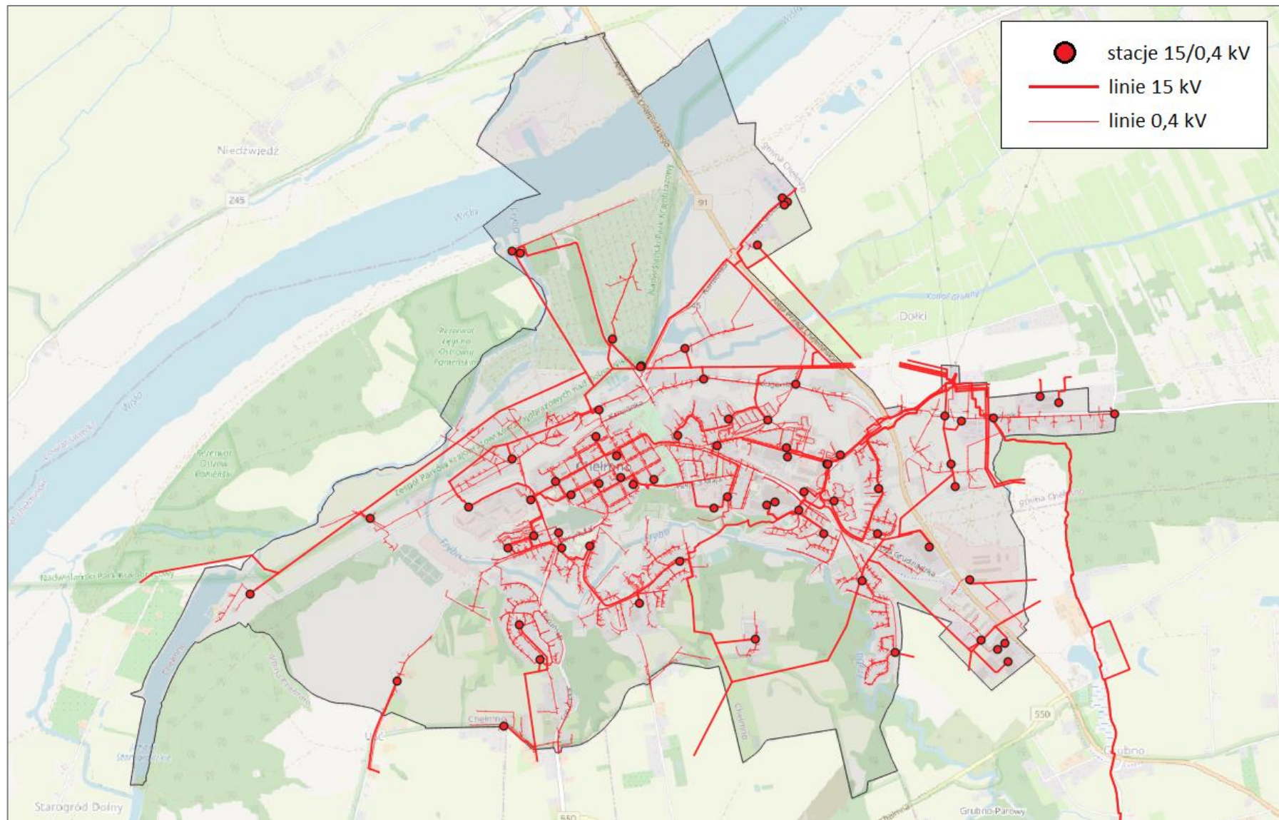
Rysunek 6. Przebieg linii elektroenergetycznych (15 kV) i (0,4 kV) wraz z rozmieszczeniem stacji transformatorowych 15/0,4 kV na terenie Chełmna
